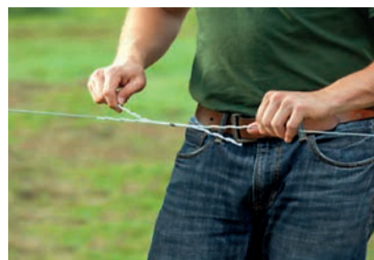
Uso de empalmes para unir alambre.
